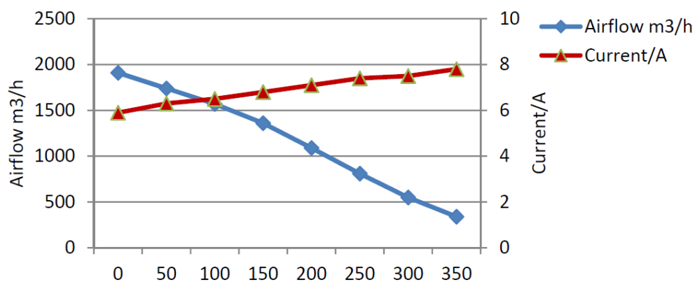
255mm 有刷轴流风机 24V DC 255mm Brushed Axial Fan
