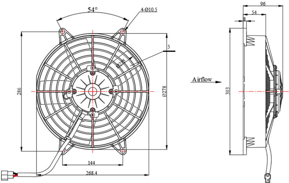
安装尺寸图 (单位: 毫米) Dimension (Unit: mm)
